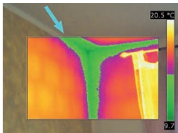
▲ Formazione di muffe all'interno di un edificio.
