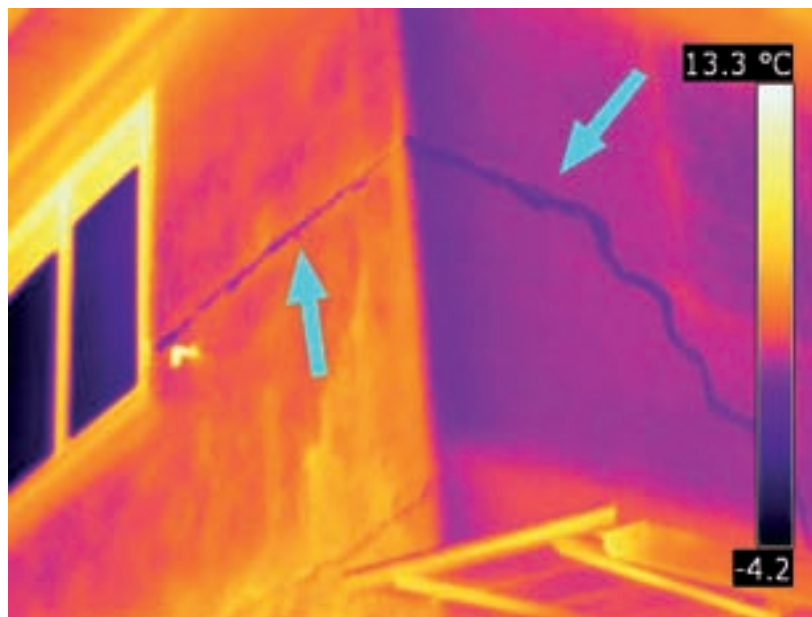
Interruzione dello strato superficiale di rivestimento.
